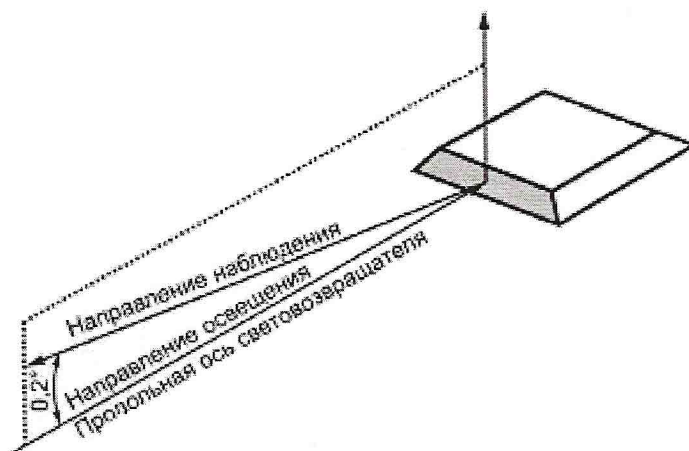
Рисунок 1 - Схема размещения световозвращателя типа КД3 при проведении фотометрических измерений при угле освещения \beta_v = 0^\circ
