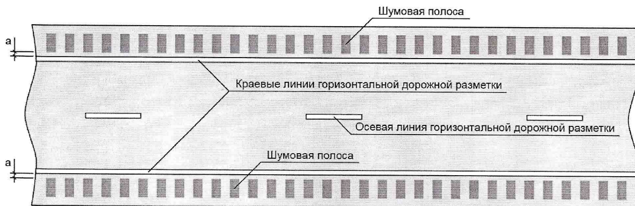
Рисунок А.3 – Пример схемы устройства продольных ШП на участке автомобильной дороги без разделительной полосы.
