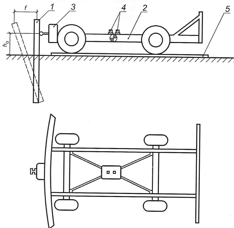
1 — стойка; 2 — ударная тележка; 3 — ударный наконечник; 4 — датчик замедления; 5 — направляющее устройство; f — величина динамического отклонения стойки; h_0 — высота удара
