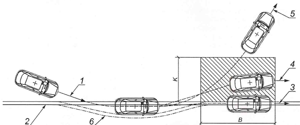
1 — траектория наезда; 2 — дорожное ограждение; 3, 4 — траектория выбега, удовлетворяющая требованиям безопасности; 5 — траектория выбега, не удовлетворяющая требованиям безопасности; 6 — линия упругого прогиба; K — ширина коридора; B — длина коридора
